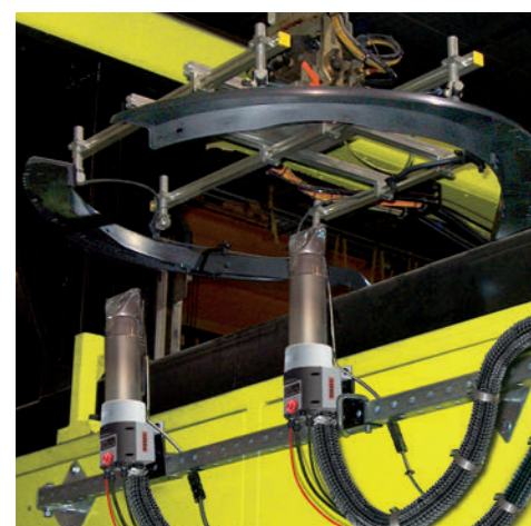
Нагреватель LHS 61 в установке очистки деталей из пластмасс направленным потоком горячего воздуха
