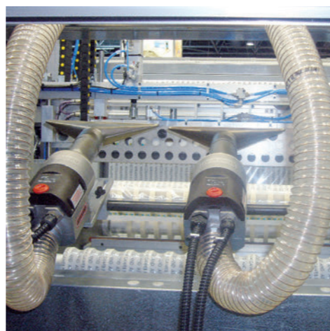
Воздухонагреватели LHS 61S с широкой щелевой насадкой в упаковочной линии
